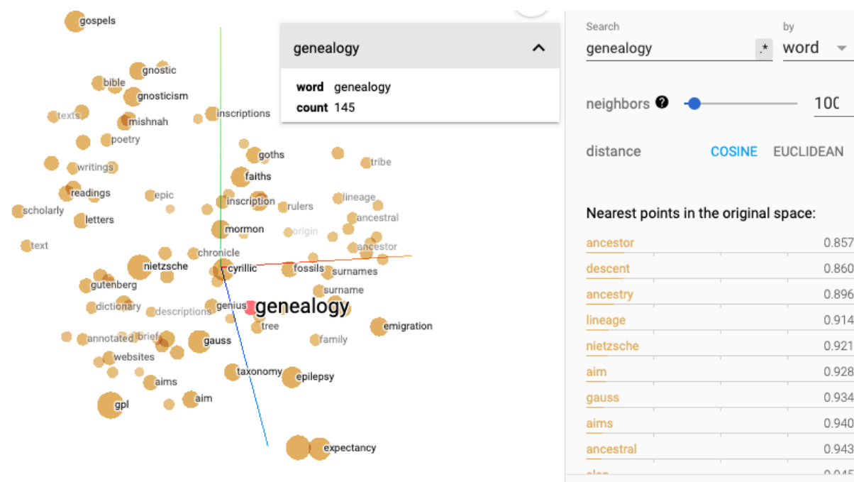
Figura 12: Mapa de incorporações de palavras produzido a partir da palavra “genealogy” gerado com a ferramenta Embedding Projector. Elaborado pela autora.
